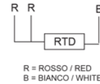
Schema di collegamento Connection diagram
